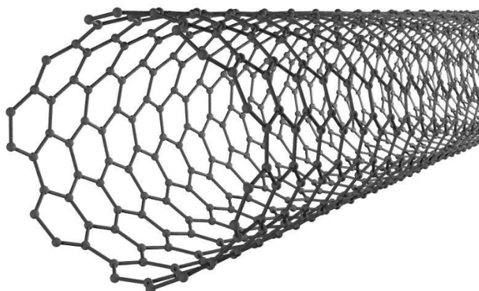
Рисунок 1. Углеродная нанотрубка
